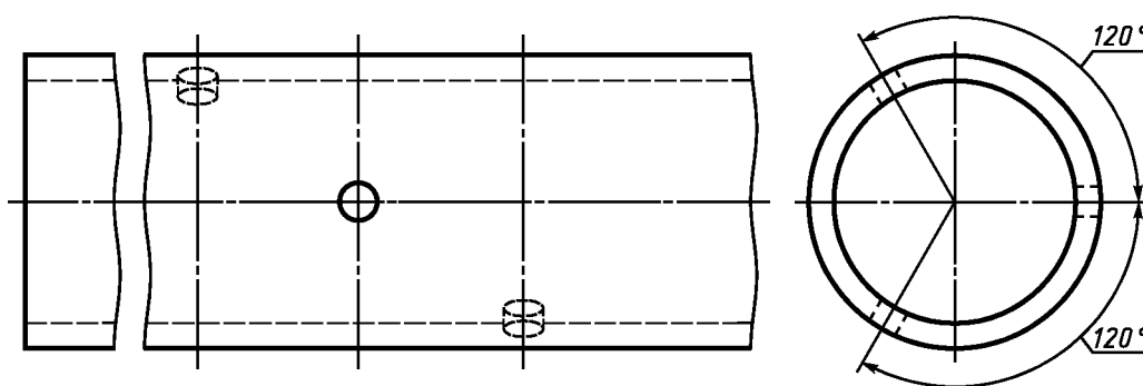
Рисунок В.1 — Эталонный образец тремя отверстиями
