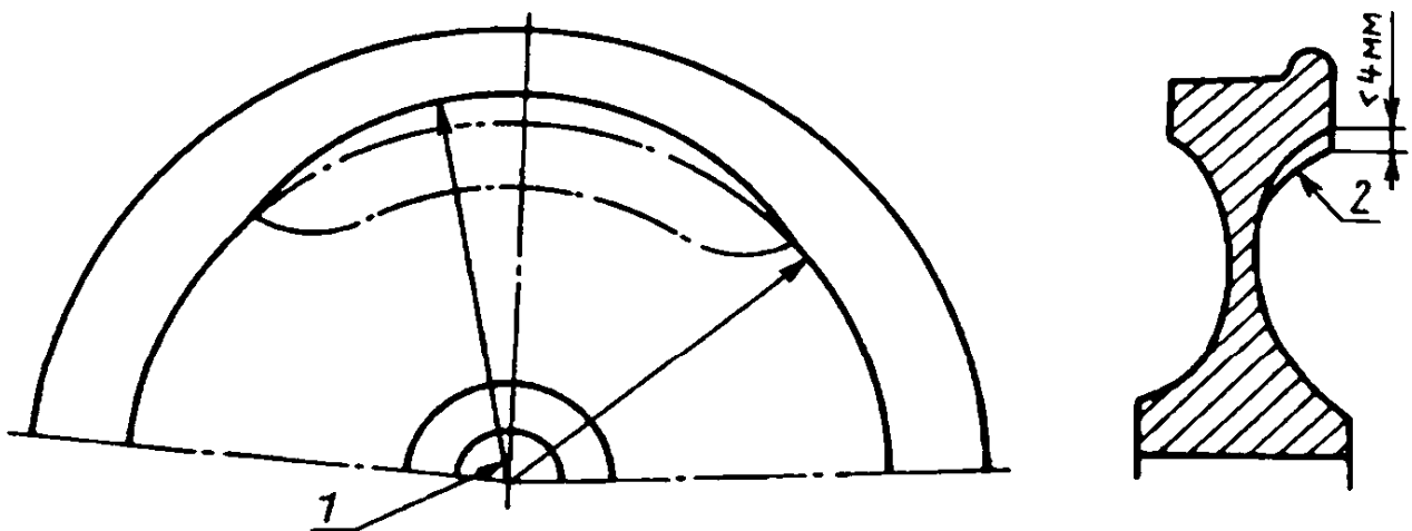
1 — дисбаланс; 2 — устранение дисбаланса
