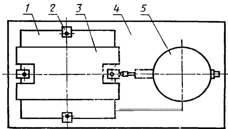
1—образец; 2—зажим; 3—прижим; 4—основание; 5—индикатор часового типа
