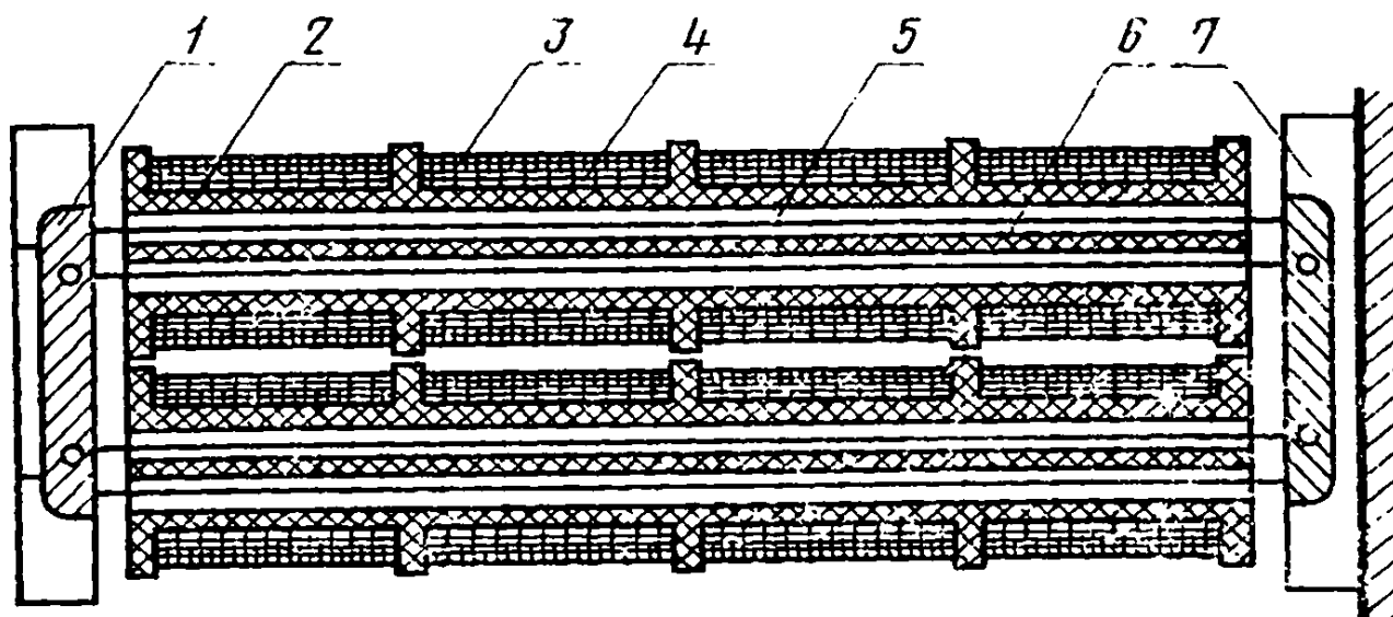
—ядро; 2—каркас соленоида; 3—намагничивающая обмотка; 4—измерительная обмотка; 5— испытываемые листы; 6—изоляционная прокладка; 7—держатель ядра
