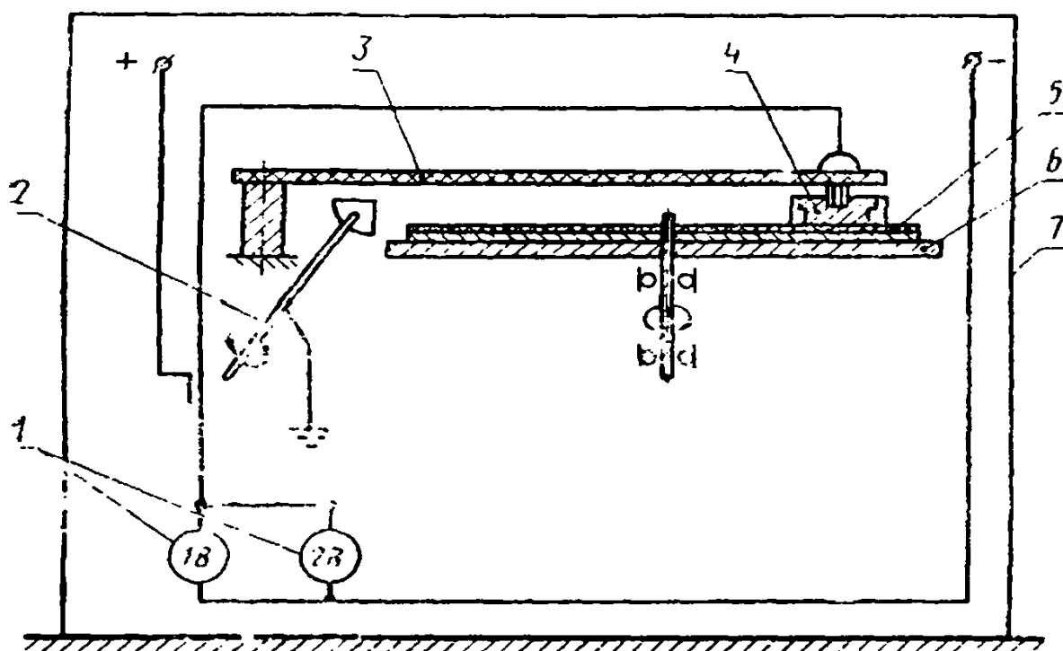
У—киловольтметры; 2—заземленный поворотный рычаг; «7—подвижный рычаг; 4—голов* на; 5—кассета с образцом; диск; 7—камера
