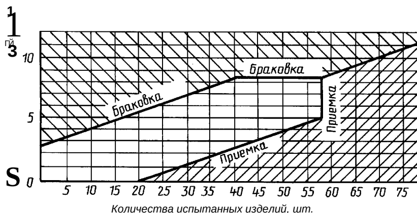
Черт. 2
