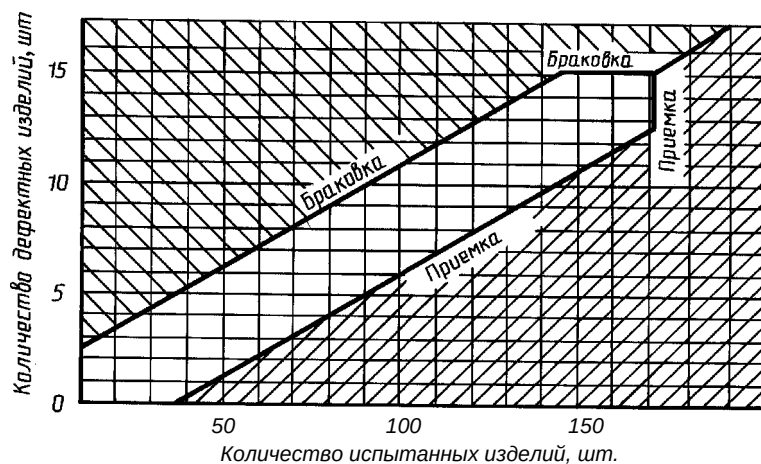
Черт. 3
