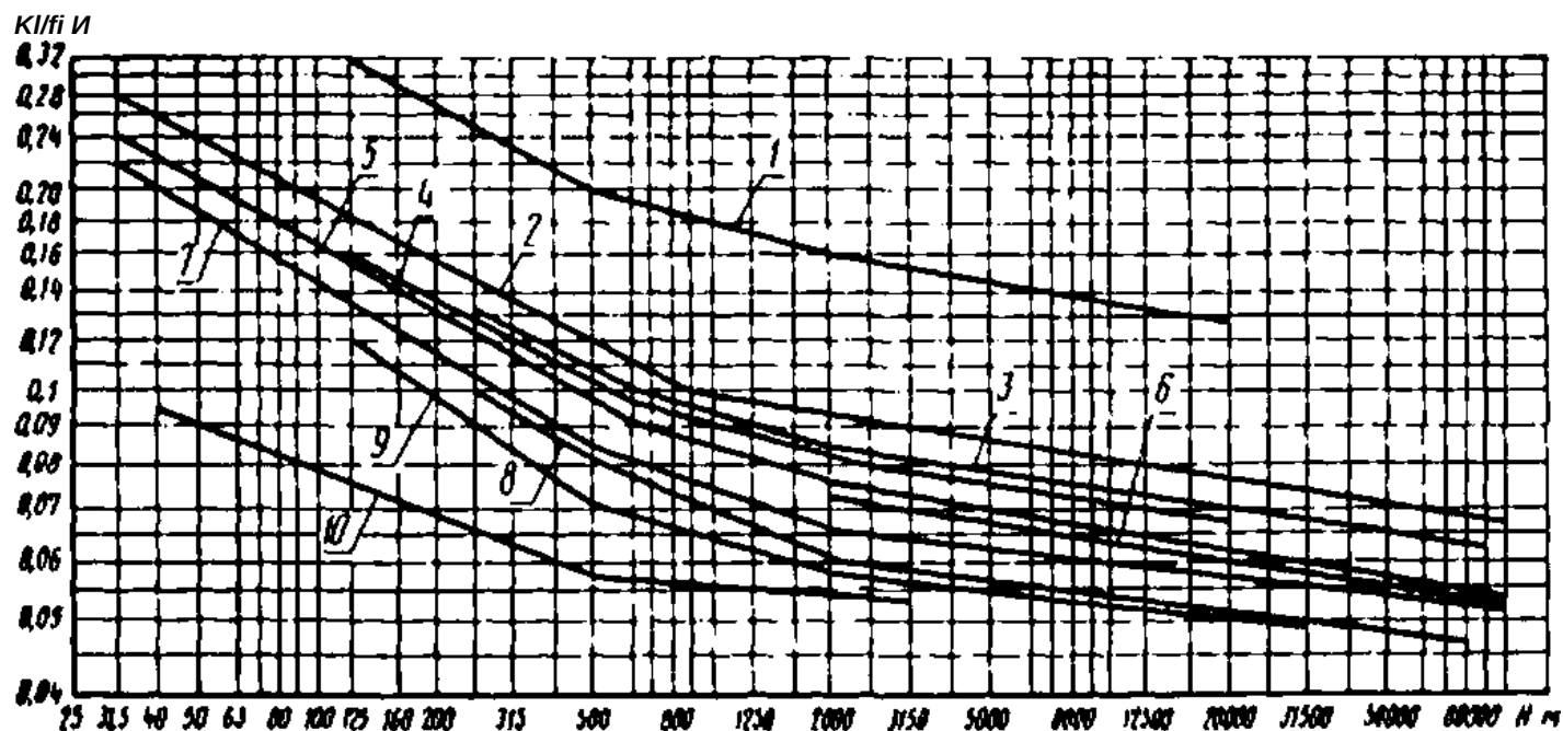
График зависимости удельной массы редукторов от крутящего момента на выходном валу
