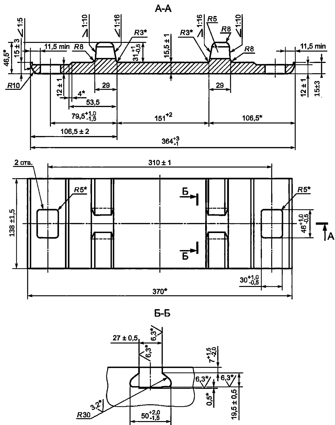
Рисунок 1 — Конструкция и размеры подкладок типа КБ 65
