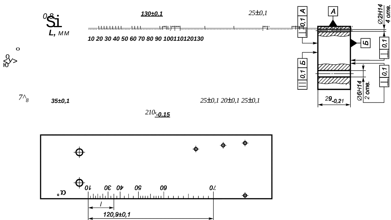
Рисунок 3 — Стандартный образец СО-2Р
