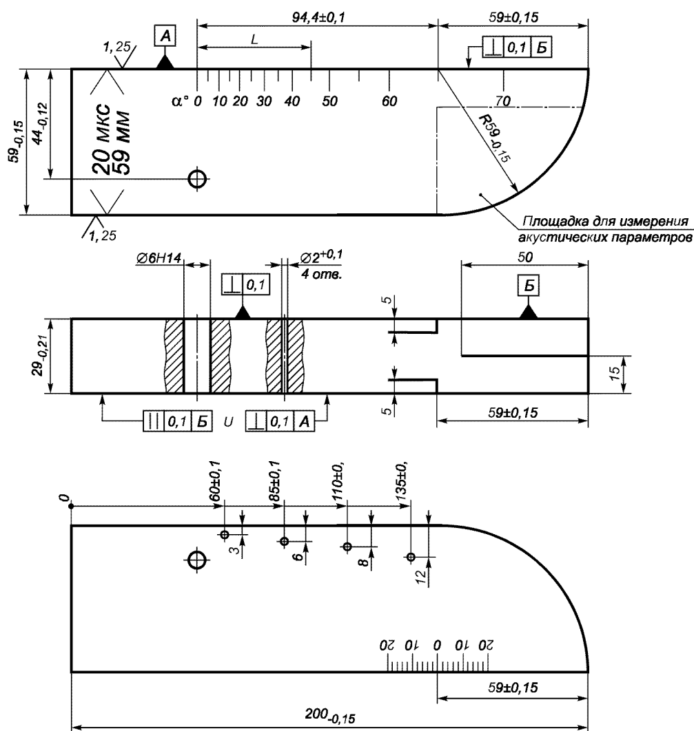
Рисунок 4 — Стандартный образец СО-ЗР
