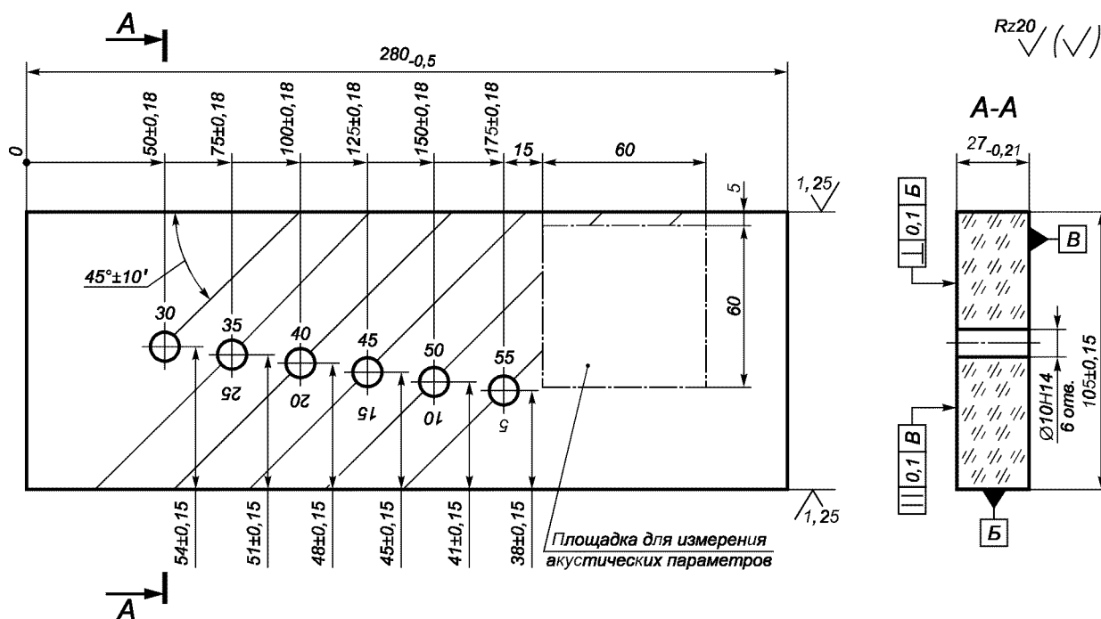
Рисунок 2 — Стандартный образец СО-1Р
