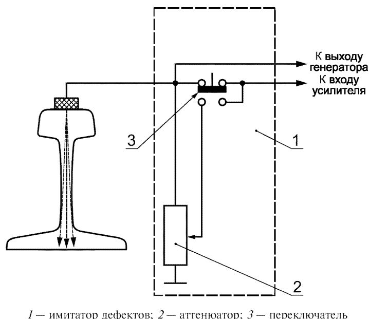
Рисунок 1 — Схема устройства для измерения условной чувствительности
