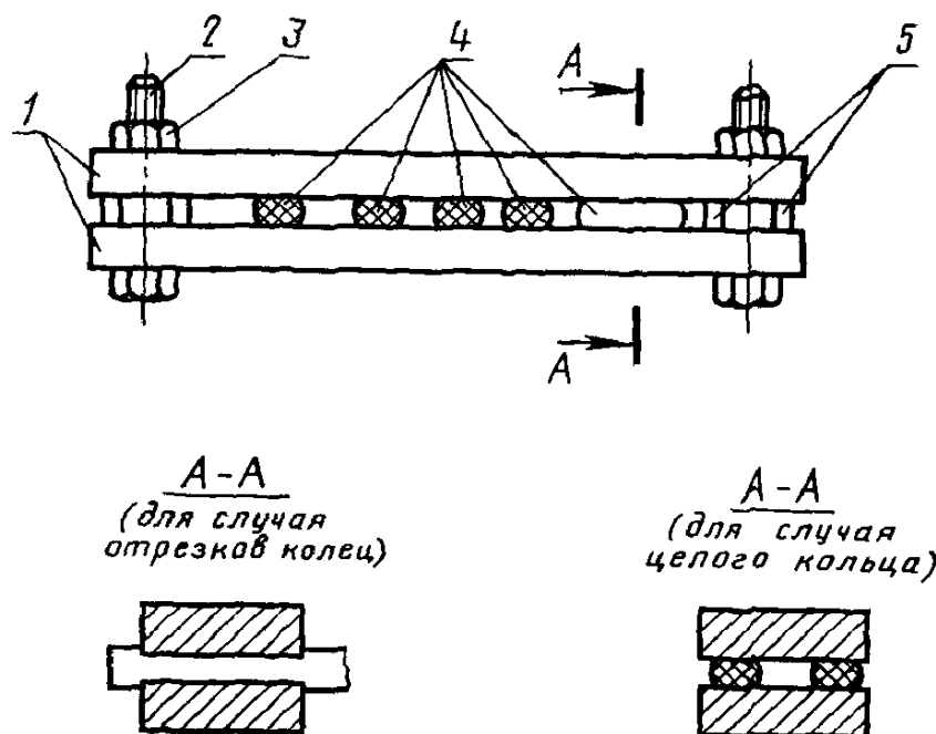
Схема струбцины с образцами
