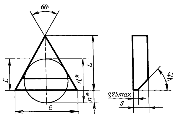
Размеры, мм
