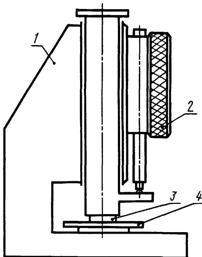
Схема прибора типа ПТШ-3
