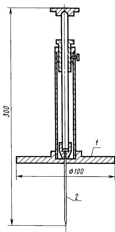
1 — диск; 2 — стержень
