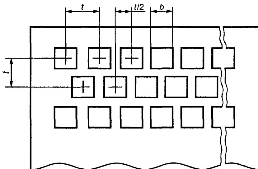
Рисунок А.1 — Схема расположения отверстий на листовых ситах
