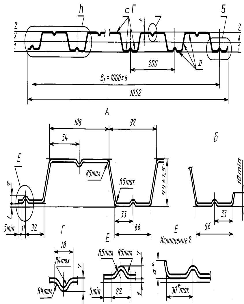
Рисунок 6 - Профилированный лист типа НС высотой 44 мм
