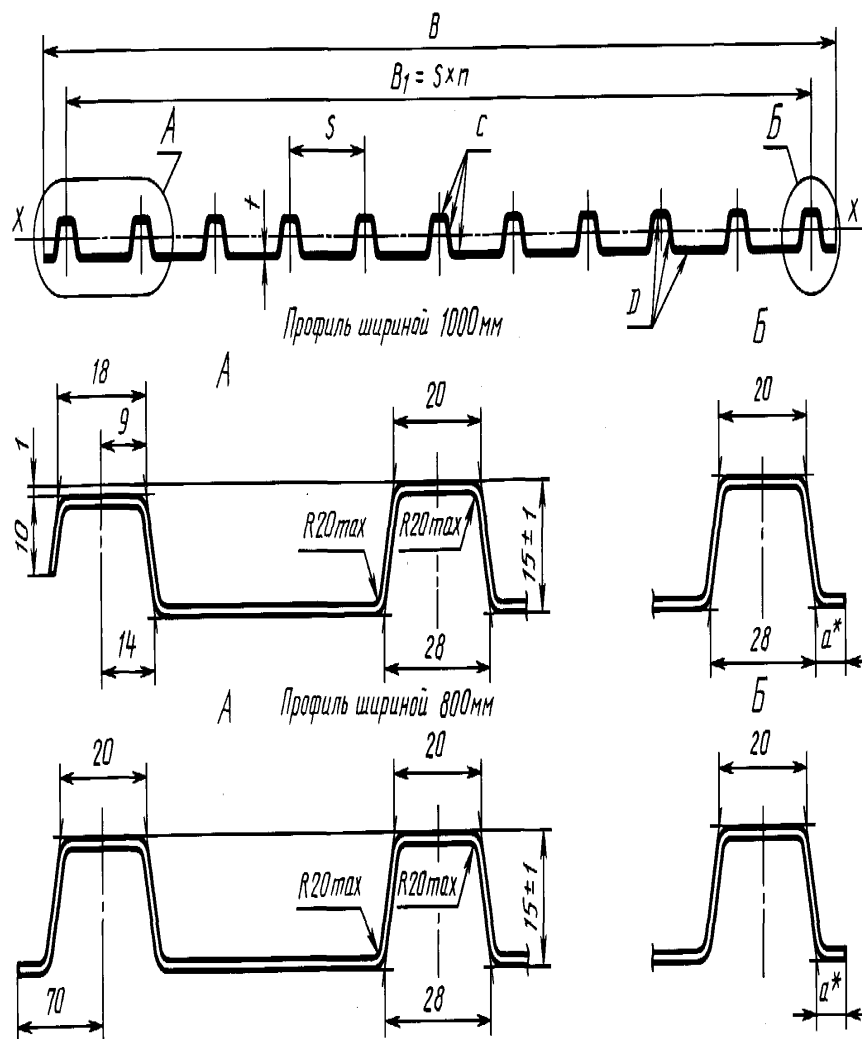
Рисунок 8 - Профилированный лист типа С высотой 15 мм
