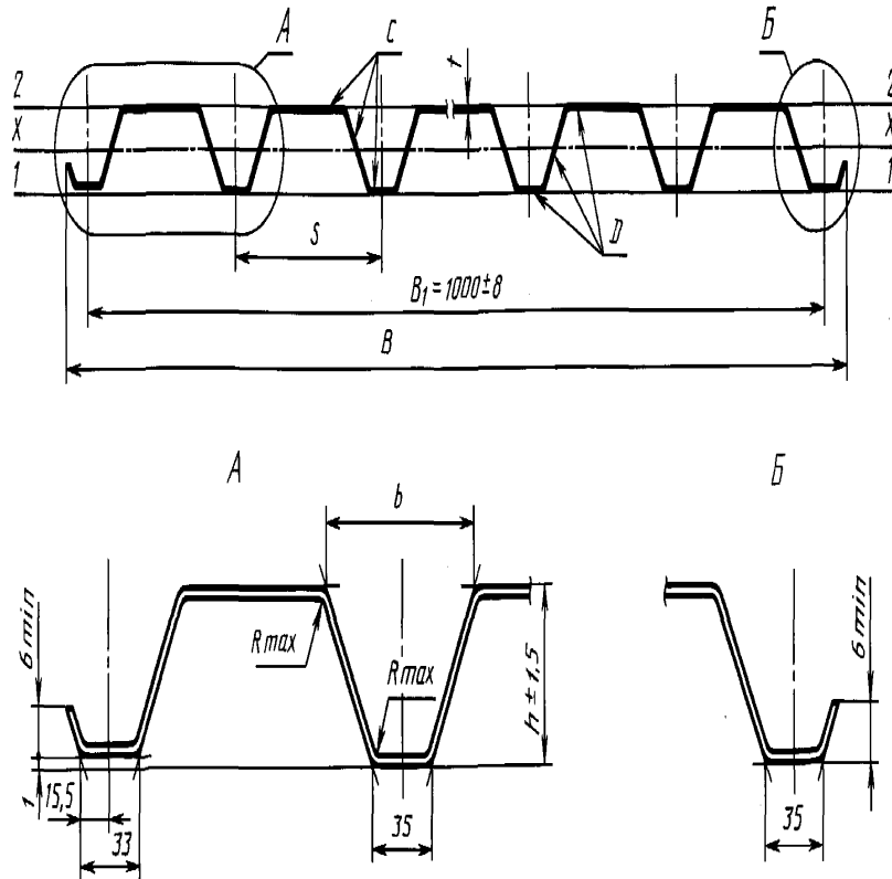
Рисунок 9 — Профилированный лист типа С высотой 21 и 44 мм
