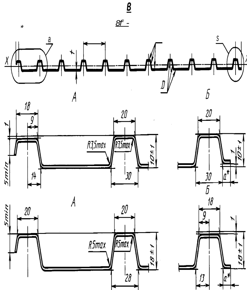
Рисунок 1 - Профилированный лист типа С высотой 10 и 18 мм
