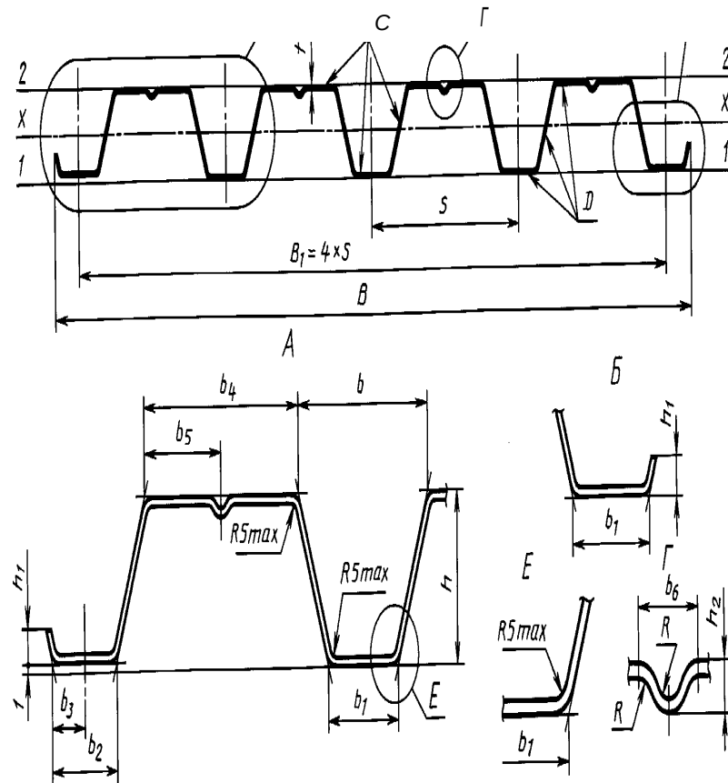
Рисунок 1 - Профилированный лист типа Н высотой 57 и 60 мм
