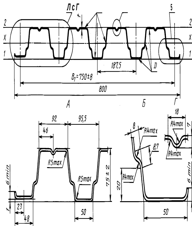
Рисунок 2 - Профилированный лист типа Н высотой 75 мм
