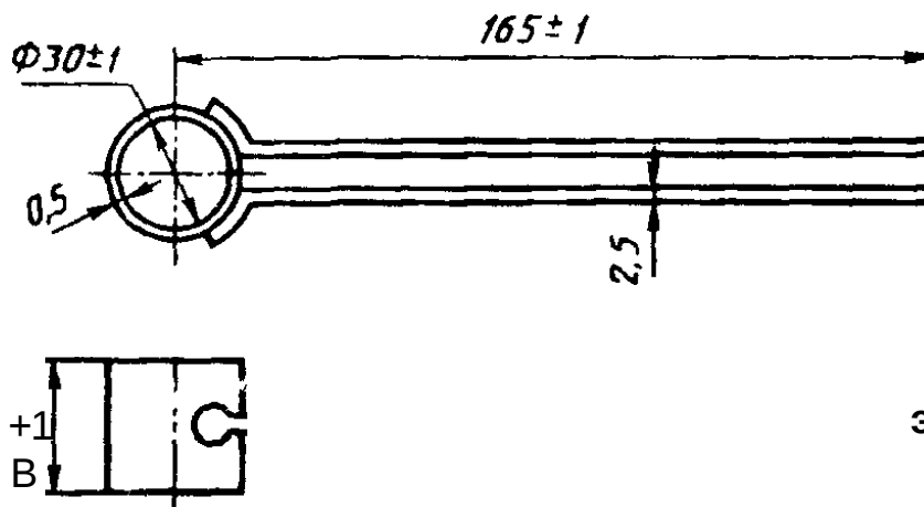
Рисунок 2 — Кольцо Ле-Шателье
