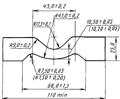
Штанцевый нож для серповидного образца
