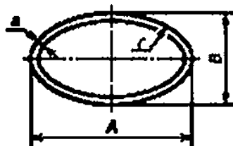
большая ось, B — малая ось; r — радиус закругления; S — толщина стенки
