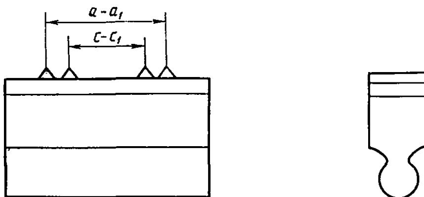
Схема штампа для нанесения меток на образцы
