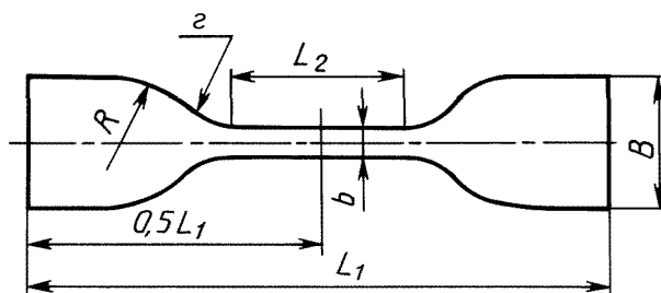
Рисунок 2 — Образец-лопатка типа 2
