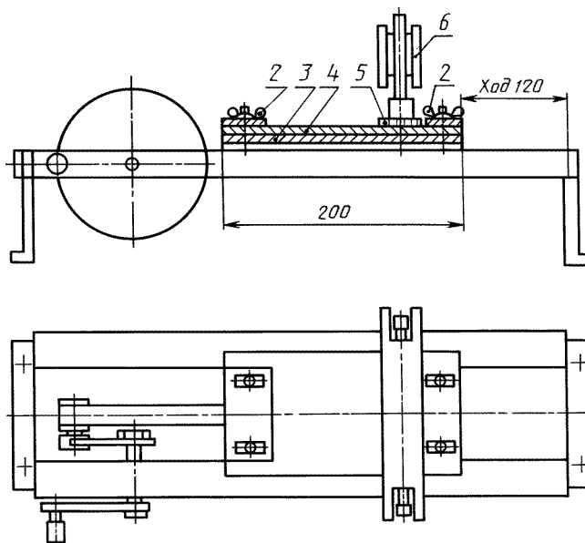
1 — рукоятка; 2 — зажимные винты; 2 — пластинка; 4 — образец; 5 — щетка; 6 — груз
