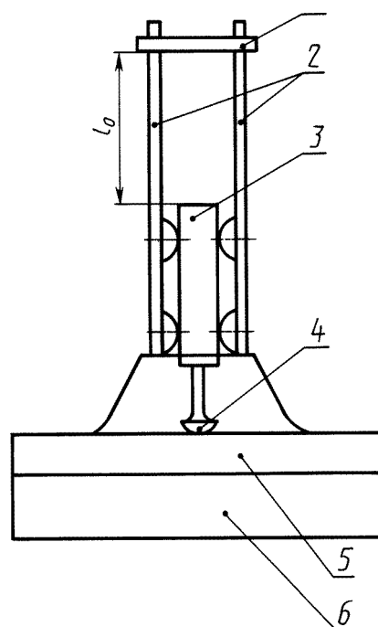
1 — ограничитель; 2 — стальные направляющие; 3 — свинцовый боек; 4 — индентор из стали Ст3 с радиусом закругления (25,0 \pm 0,3) мм; 5 — испытуемый образец; 6 — подложка
