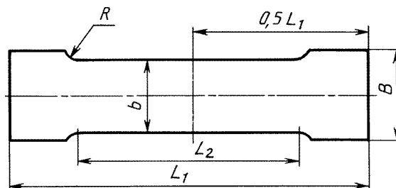
Рисунок 1 — Образец-лопатка типа 1
