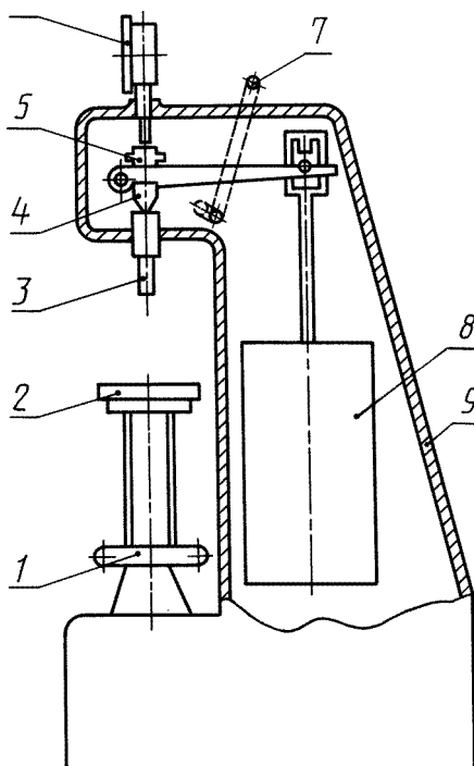
1—гайка-маховик; 2—подъемный столик; 3—индентор; 4—призма рычага основной нагрузки; 5—шпindel с грузом предварительной нагрузки; 6—отсчетное устройство; 7—рукоятка приложения и снятия основной нагрузки; 8—грузы для основной нагрузки; 9—корпус
