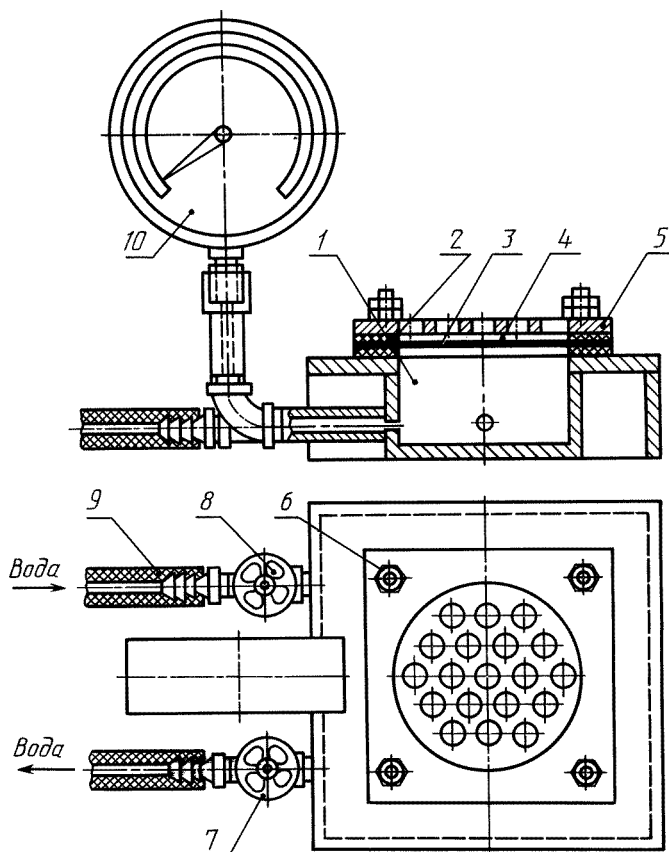
1 — рабочая камера; 2 — резиновые прокладки; 2 — образец; 4 — контактная сетка; 5 — прижимная плита; 6 — зажимные винты; 7, 8 — краны; 9 — резиновая трубка, соединяющая с водопроводом; 10 — манометр
