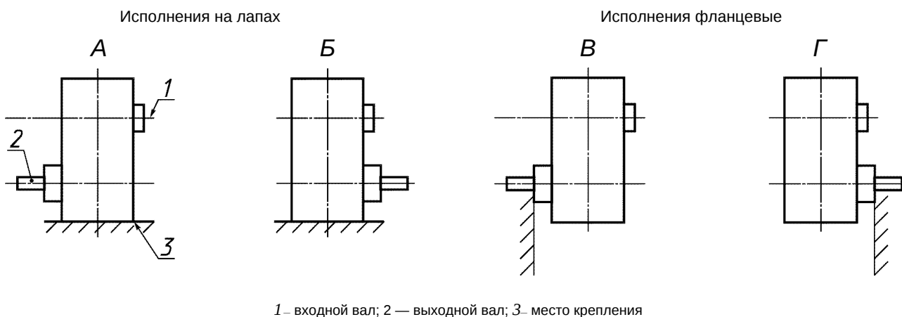
Рисунок А. 1 — Варианты сборок
