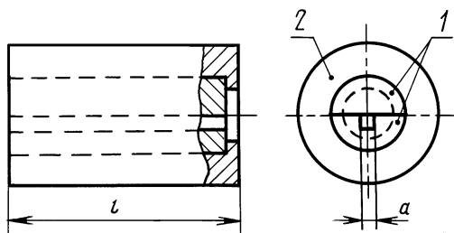
1 — полуматрица; 2 — обойма
