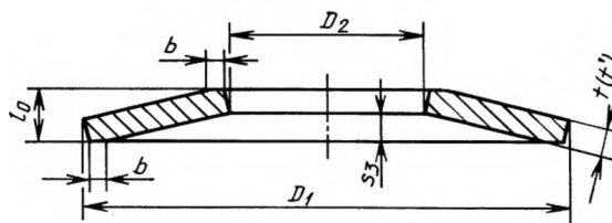
Пружина типа 2
