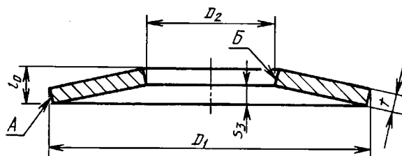
Пружина типа 1
