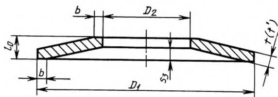
Пружина типа 4
