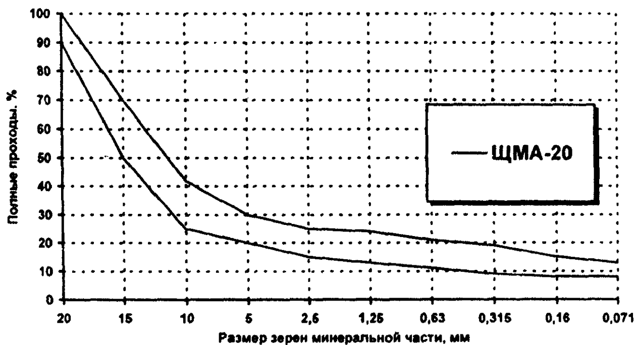
Рисунок Б.3 — Зерновой состав минеральной части ЩМА-20
