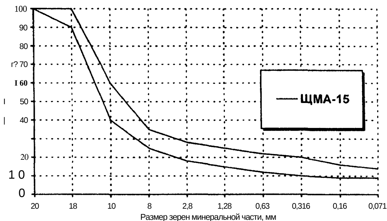
Рисунок Б.2 — Зерновой состав минеральной части ЦМА-15
