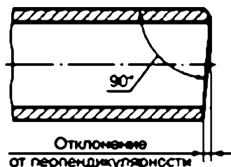
Рисунок 3 — Неперпендикулярность
