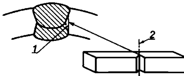
1 — материал, отбираемый для изготовления образца с V-образным надрезом для испытаний на ударную вязкость в зоне термического влияния (HAZ) сварного шва вблизи линии плавления. 2 — ось надреза на образце для испытания на ударный изгиб
