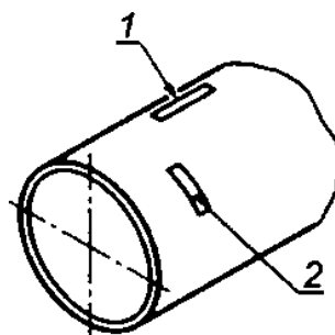
1 — L — продольная проба, 2 — Т — поперечная проба
