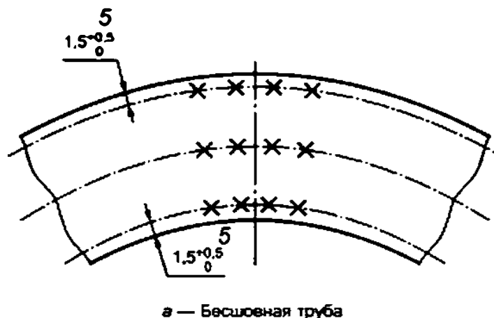
Рисунок А.1 — Места контроля твердости
