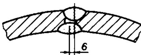
д — Смещение валиков сварного шва на трубах КОС
