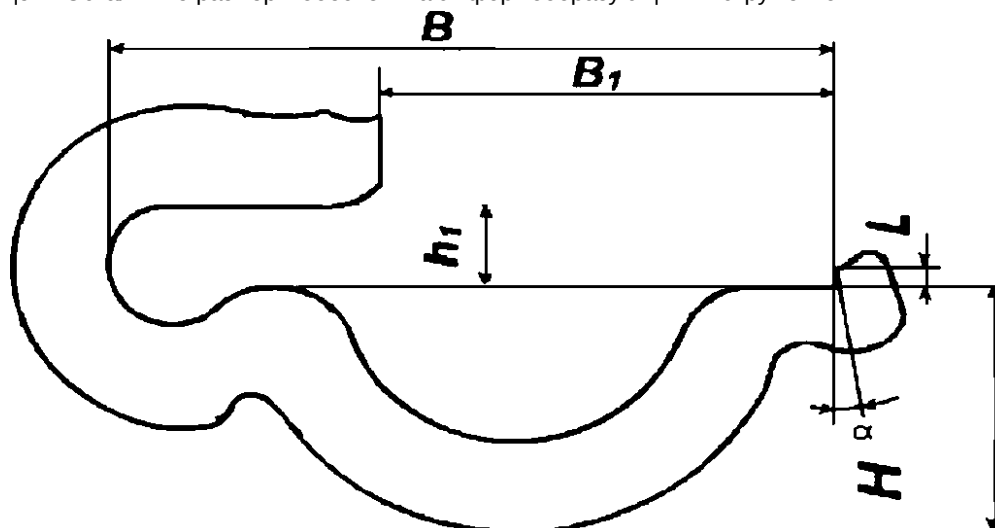
Рисунок 1 - Конструкция пружинного противоугла в первом исполнении для железнодорожного пути на деревянных шпалах
