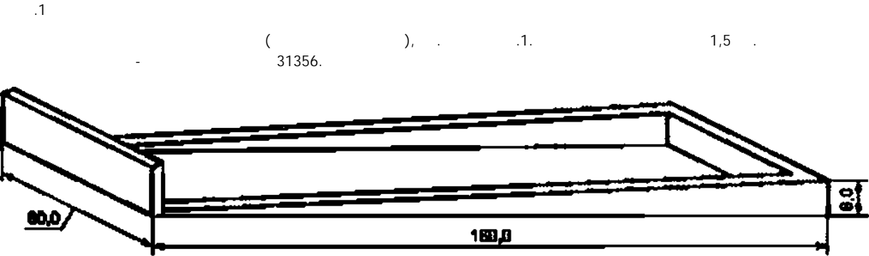
Рисунок А.1 — Форма для изготовления образцов при определении стойкости к образованию трещин
