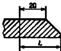
Рисунок А — Присоединительный конец под приварку
