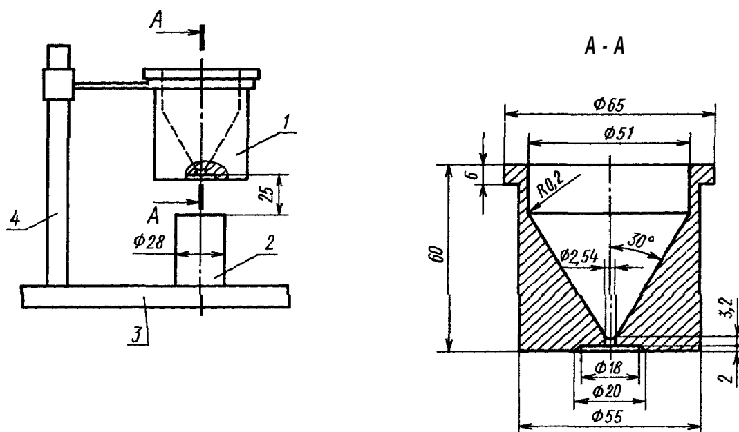
1 — воронка, изготовленная из парамагнитного материала твердостью 140 НВ (сталь марки Ст40Х), с калиброванным выходным отверстием диаметром 2,54 мм; 2 — цилиндр-уловитель; 3 — штатив; 4 — стойка
