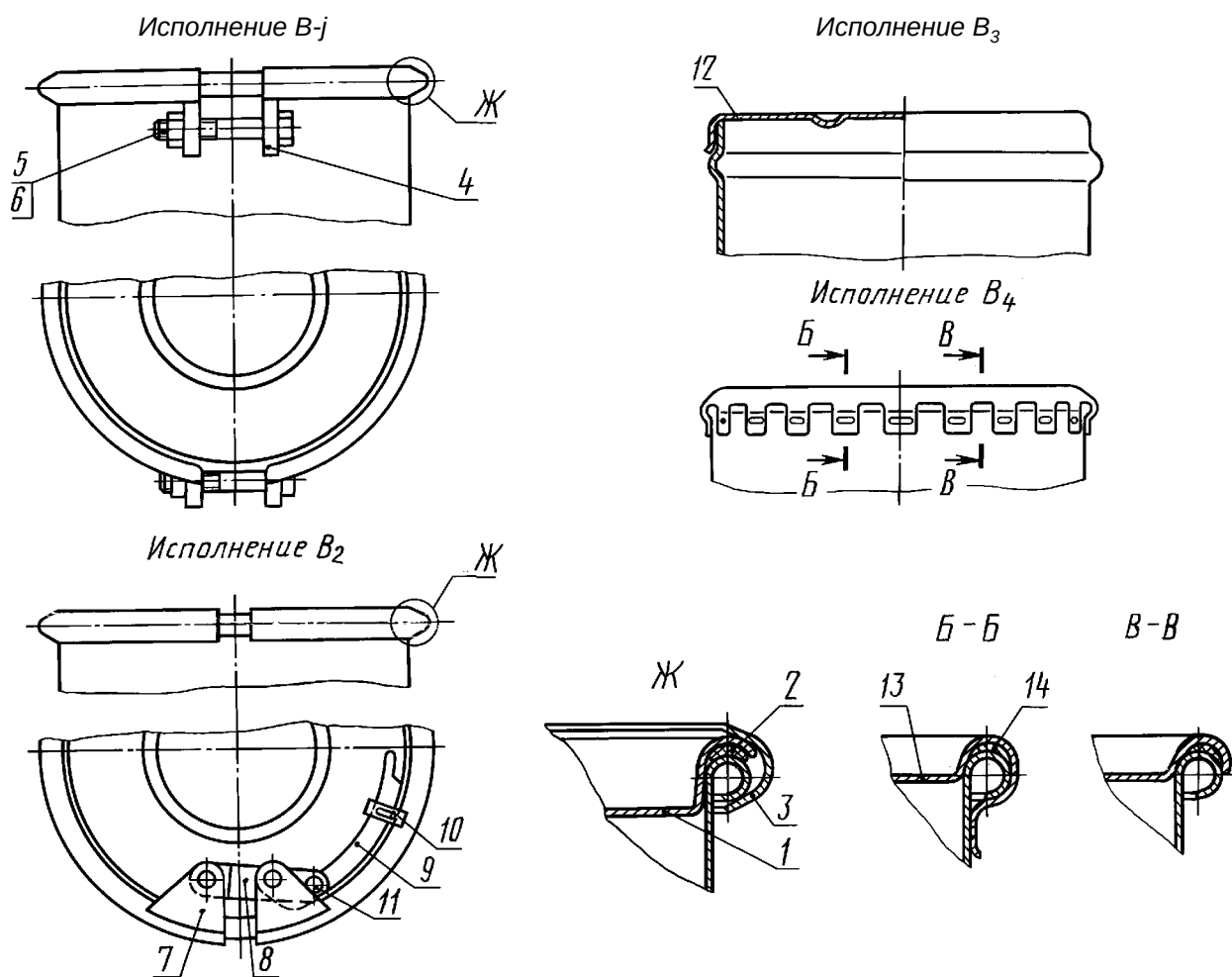
1, 12, 13 — верхние днища; 2 — прокладка; 3 — стяжной обруч; 4 — косынка; 5 — болт М12 ГОСТ 7798—70; 6 — гайка М12,4 ГОСТ 5915—70; 7—косынка; 8 — тяга; 9 — рычаг; 10— ушко; 11 — заклепка 5 ГОСТ 10299—80; 14 — прокладка
