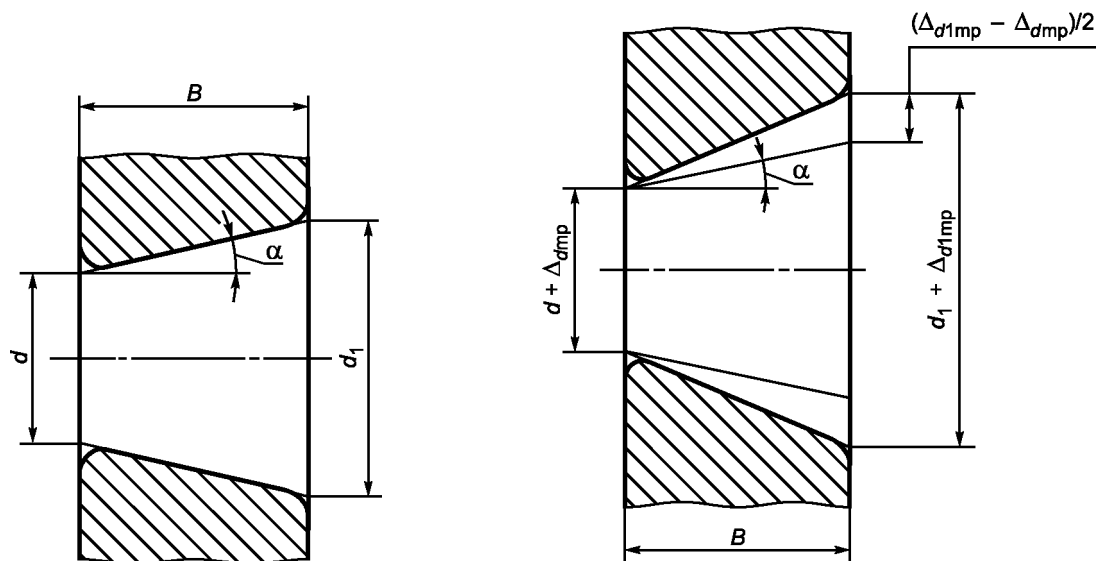
Рисунок 4 — Номинальное коническое отверстие Рисунок 5 — Действительное коническое отверстие
