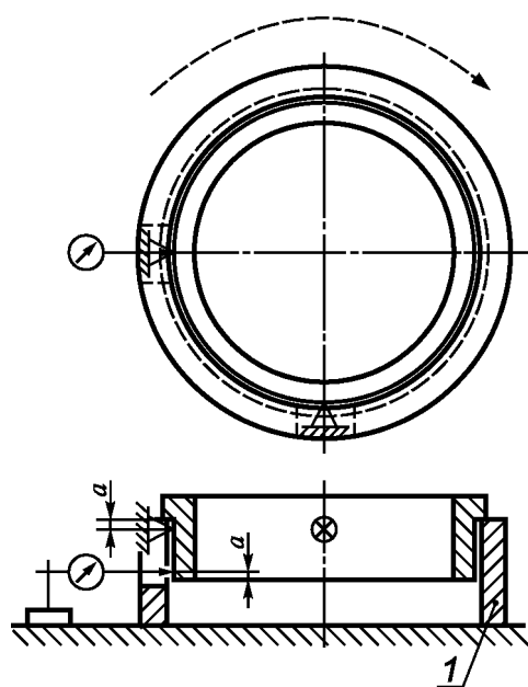
1 — кольцеобразная цилиндрическая опора a — предел зоны измерений
