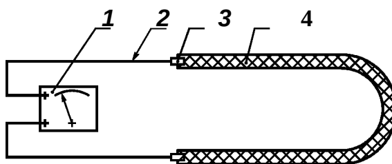
1 — измерительный прибор; 2 — проводник; 3 — электрод; 4 — рукав
