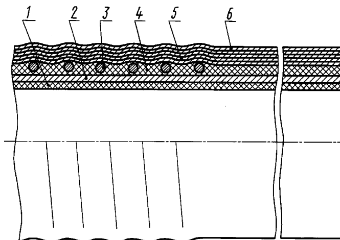
Схема конструкции рукава
