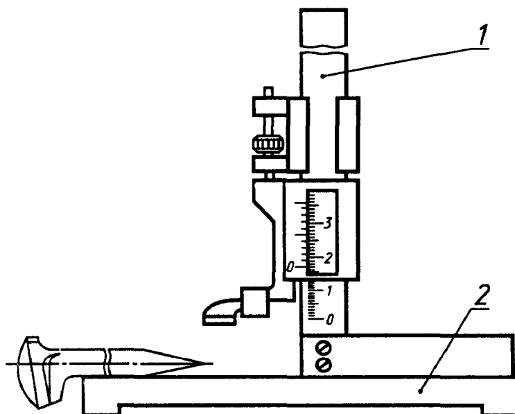
1 — штангенрейсмасс типа ШР-250—0,05; 2 — основание
