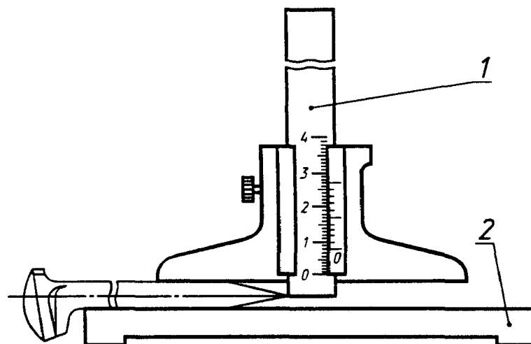
1 — штангенглубиномер типа ШГ-160; 2 — основание
