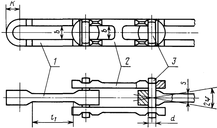
1 — внутреннее звено; 2 — наружное звено; 3 — валик
