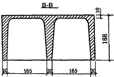
Рисунок Б.1 — Камень стеновой рядовой
