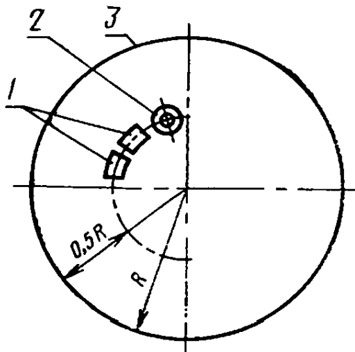
Схема вырезки образцов для механических испытаний
