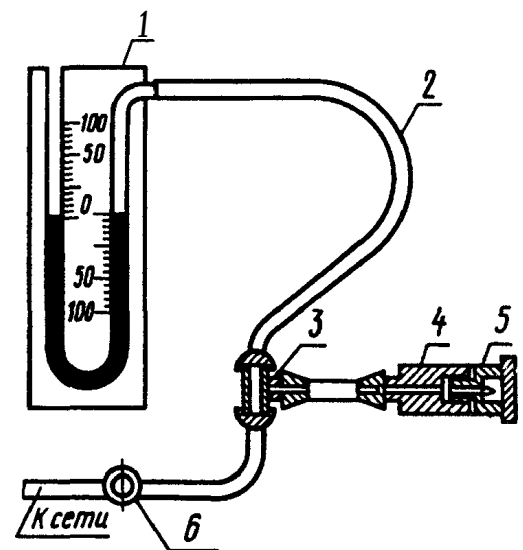
1 — ртутный манометр; 2 — шланг; 3 — тройник; 4 — патрон; 5 — пробка; 6 — кран
