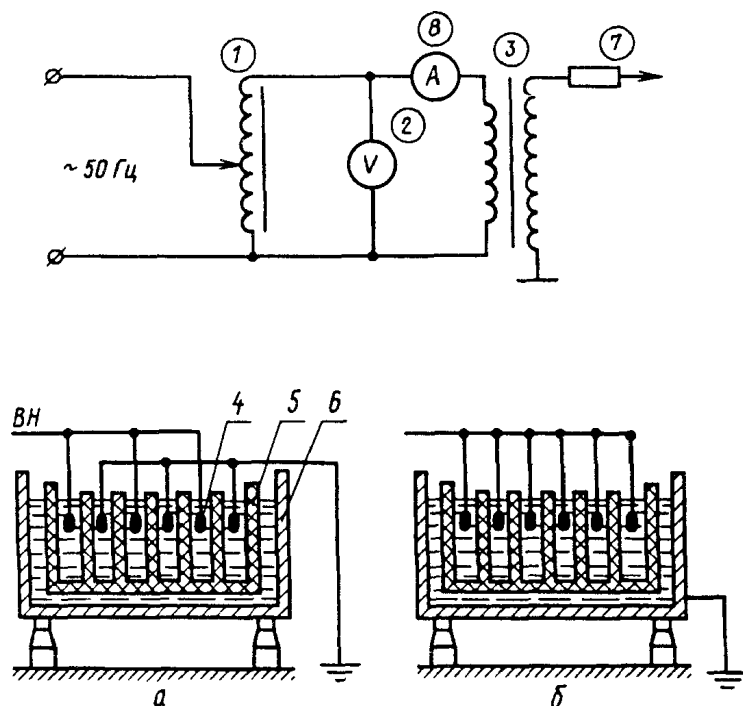
а — схема подключения электродов к источнику высокого напряжения при испытании перегородок моноблока; б — схема подключения электродов к источнику высокого напряжения при испытании корпуса моноблока. 1 — автотрансформатор регулировочный; 2 — вольтметр; 3 — высоковольтный трансформатор — источник высокого напряжения; 4 — электроды, 5 — моноблок; 6 — резервуар, 7 — защитное сопротивление; 8 — амперметр.
