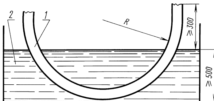
R — радиус изгиба; 1 — образец кабеля; 2 — соляная ванна
