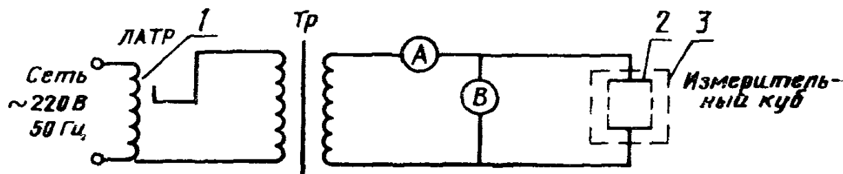
1 — лабораторный регулировочный трансформатор (ЛАТР); 2 — электрод; 3 — измерительный куб
