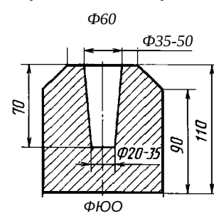
Изложница с формой усеченного конуса
