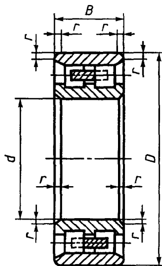
Тип 282000
