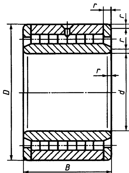
Тип 452000
