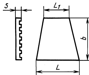
Черт. 4
